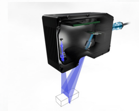
Scheimpflug Lens
